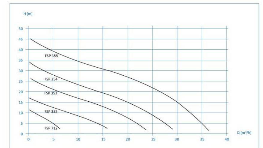
FSP系列选型表
