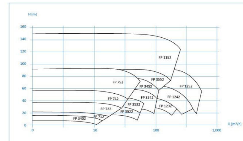
FP系列选型表 转速n=2900rpm
